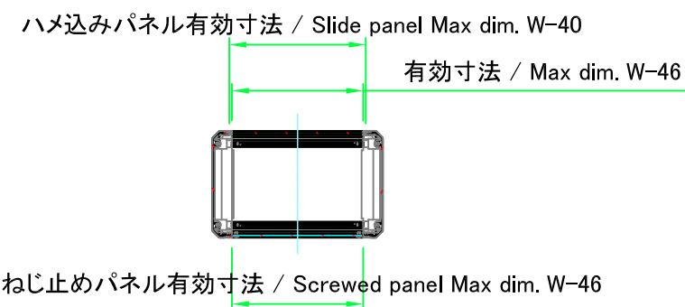
A-A ( 1 : 8 )
