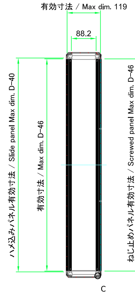
C : フレーム拡大図 / Frame cross-section
